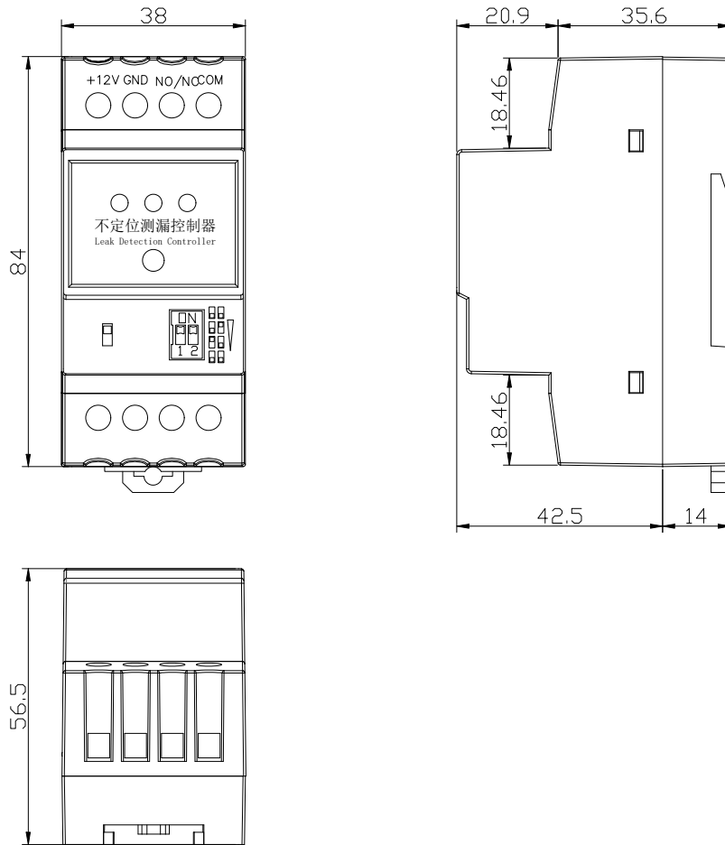
图 1 尺寸图
