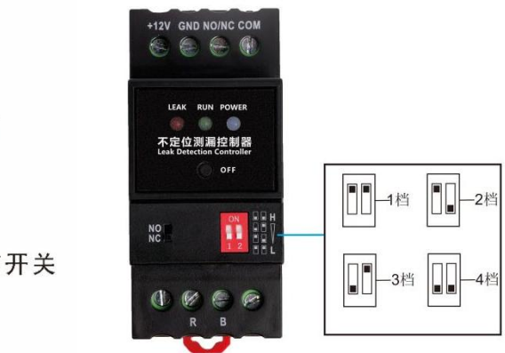
图 3 灵敏度档位按键调节示意图
