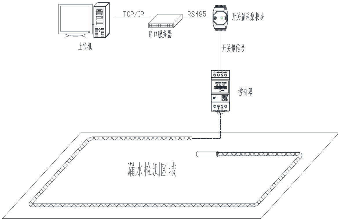
图 4 系统拓扑图
